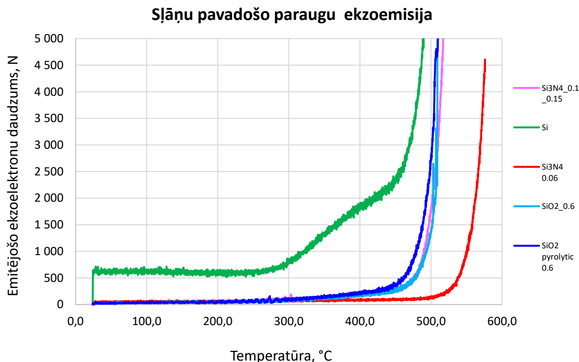
2. attēls. Slāņu pavadošos paraugu Si , SiO_2 0,6\mu m , SiO_2 0,6\_Pyrolytic 0,6\mu m , Si_3N_4 0,06\mu m un Si_3N_4 0,1 - 0,15\mu m elektronu ekzoemisijas mērījumi.
